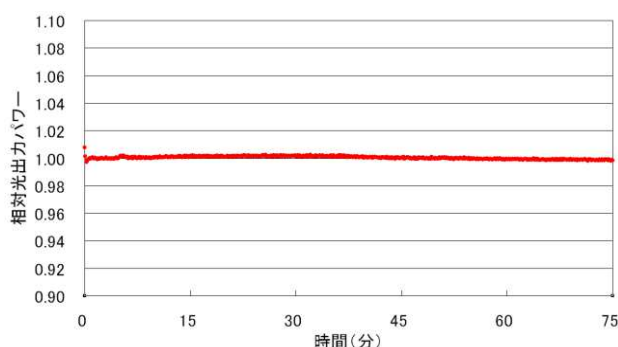
出力パワー安定度例(850nm10mW 室温下)
